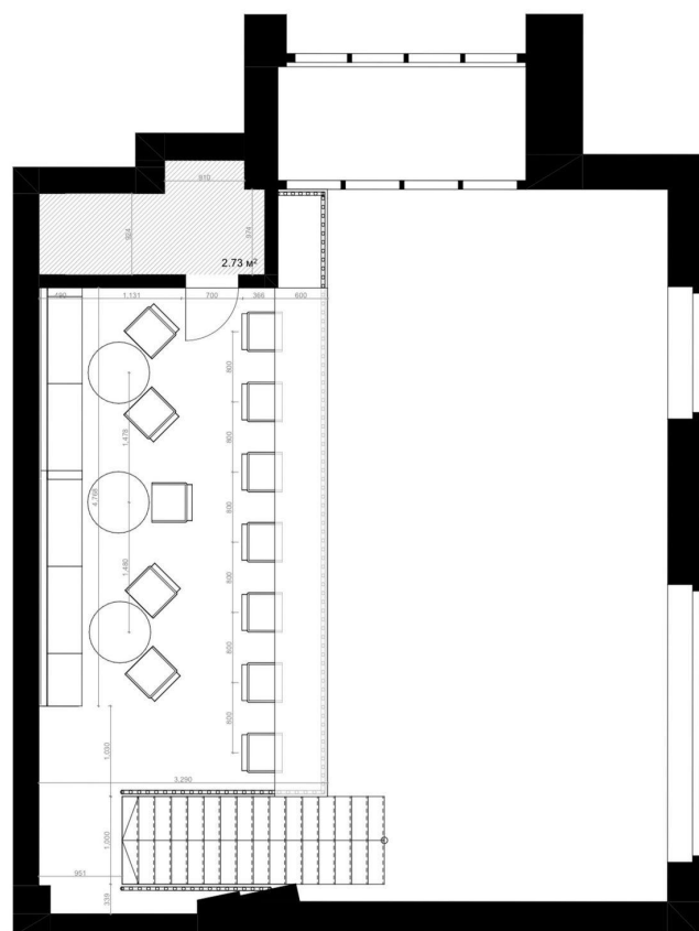
Расстановка мебели 2 этаж
